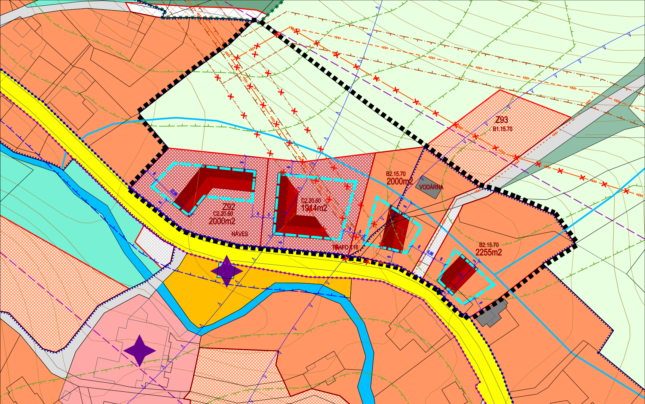
MNÍŠEK-FOJTKA, ZASTAVOVACÍ STUDIE PLOCHY Z92+DALŠÍCH, ING.ARCH.PLAŠIL, 06/17 KOORDINAČNÍ VÝKRES M 1:1000
